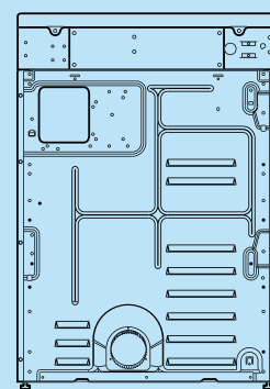
SD10 Rückansicht
