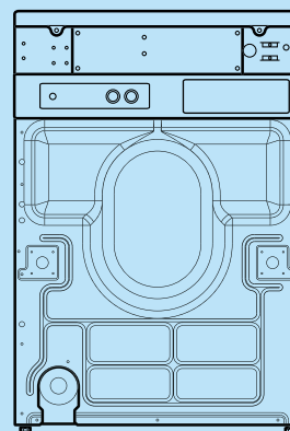
SD10 Rückansicht
